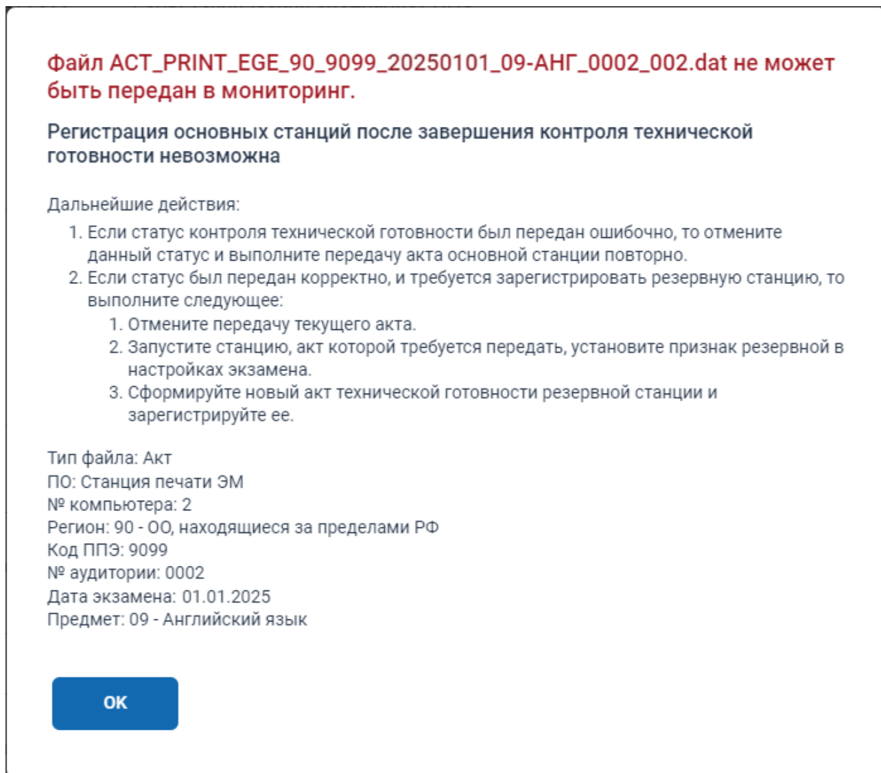
Рис. 5.12. Передача запрещена. Регистрация основных станций после завершения КТГ запрещена
