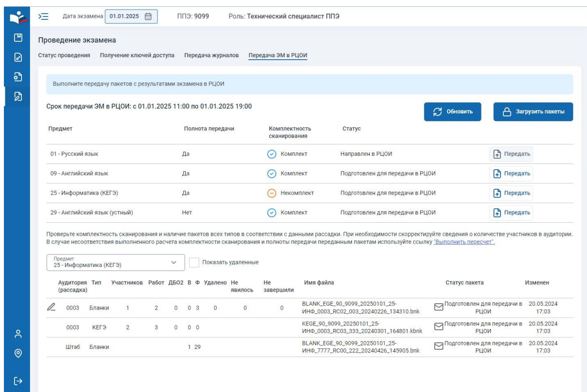
Рис. 3.81. Передача пакетов по русскому языку завершена. Пакеты доступны для скачивания в РЦОИ
