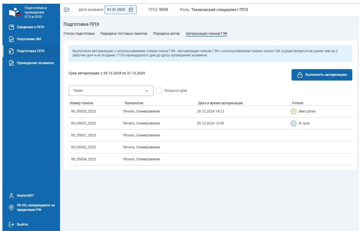
Рис. 3.38. Страница «Авторизация членов ГЭК»
