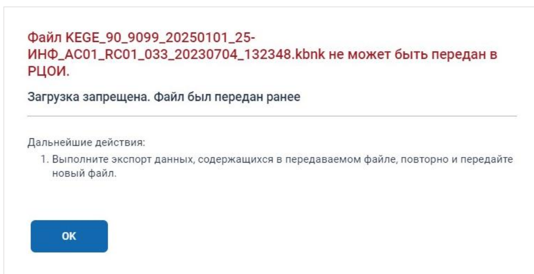
Рис. 5.29. Сообщение при попытке загрузки ранее переданного файла пакета
