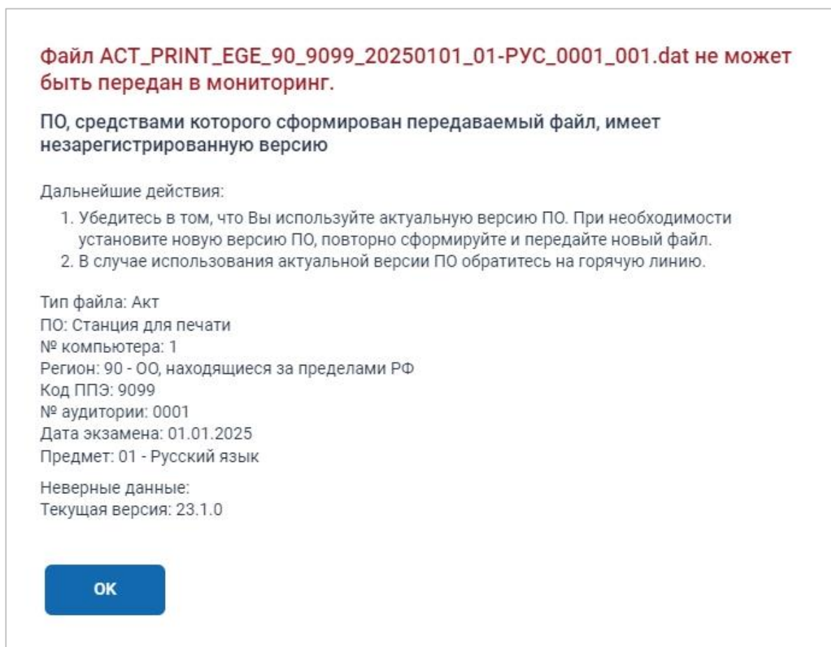
Рис. 5.6. Передача запрещена. Незарегистрированная версия станции
