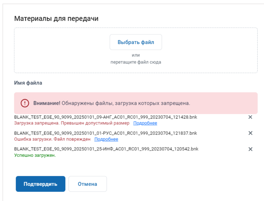
Рис. 3.24. Окно «Материалы для передачи». Результат проверки файлов, отобранных для передачи
