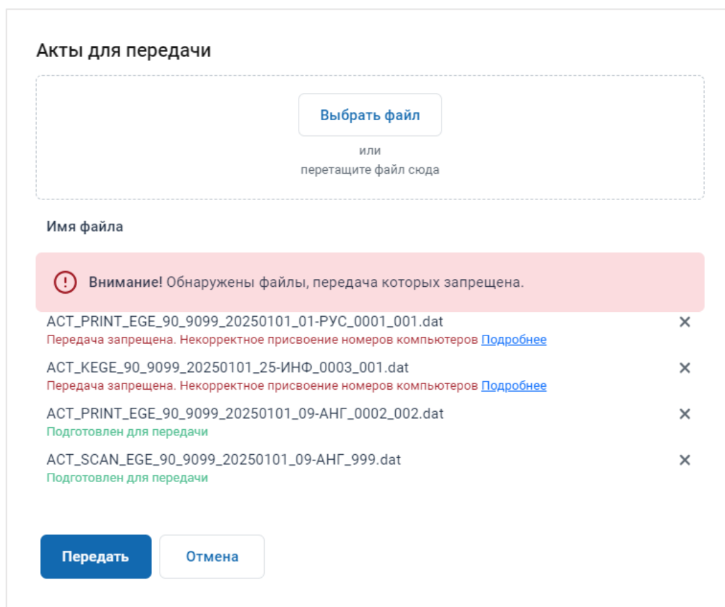
Рис. 3.34. Окно «Акты для передачи». Результат проверки файлов, отображенных для передачи
