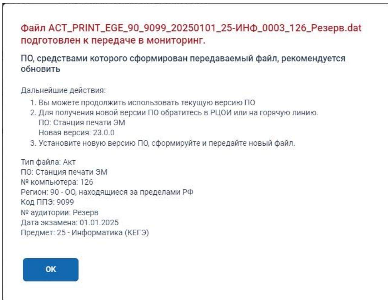
Рис. 5.8. Рекомендовано обновление ПО
