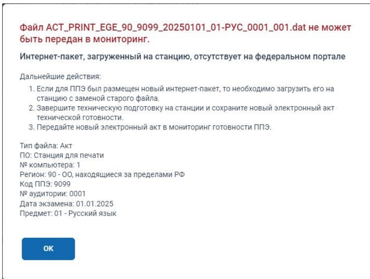
Рис. 5.5. Передача запрещена. Интернет-пакет отсутствует на федеральном портале
