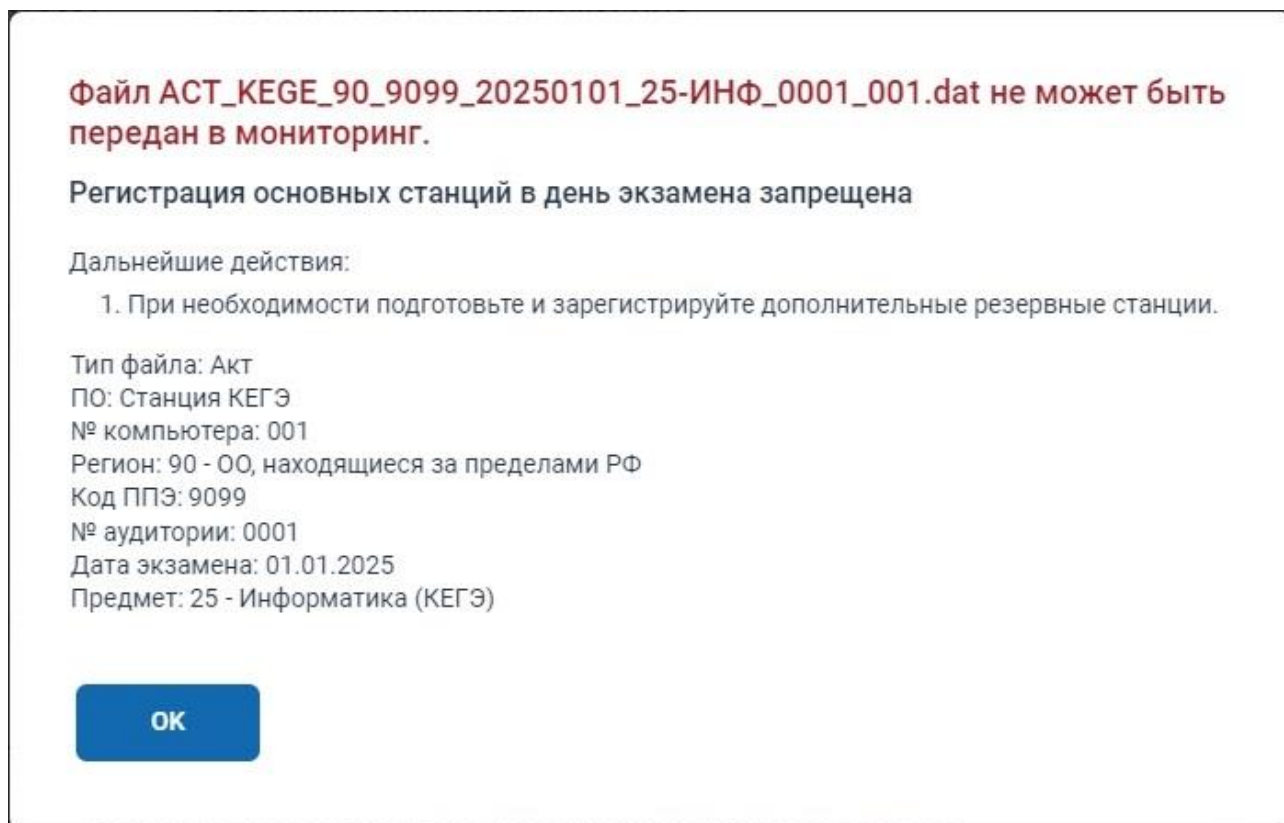
Рис. 5.13. Передача запрещена. Регистрация основных станций в день экзамена запрещена
