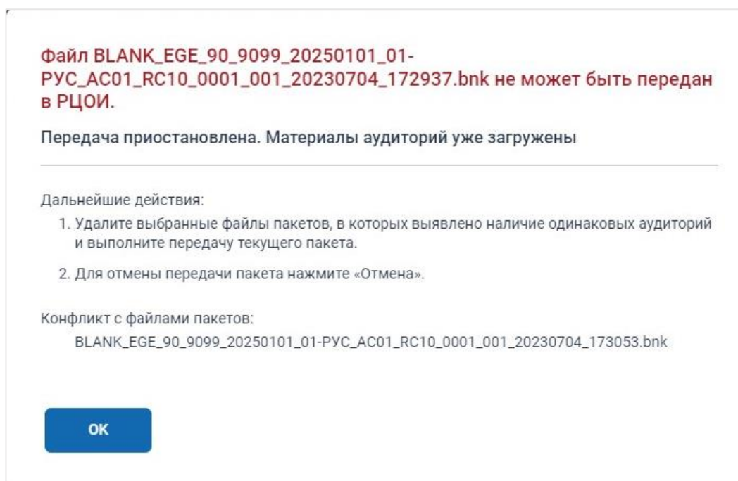
Рис. 5.31. Сообщение при попытке загрузки нескольких файлов пакетов из одной аудитории
