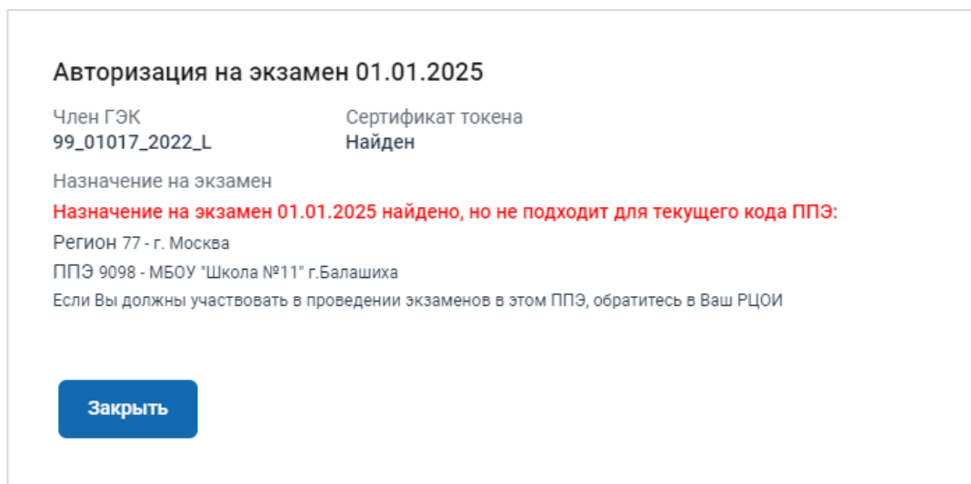
Рис. 5.17. Нештатная ситуация: Член ГЭК назначен на экзамен в другом ППЭ
